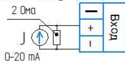
Датчик тока
