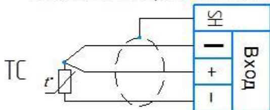
Термосопротивление с компенсацией сопротивления линии
