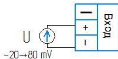
Датчик напряжения
